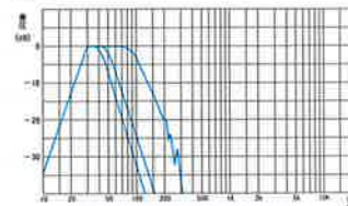
■SL-10音圧周波数特性
