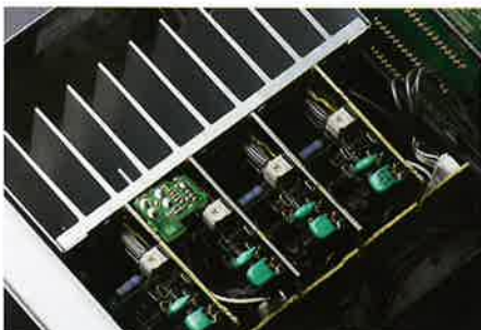
モノリス・コンストラクション・パワーアンプ
